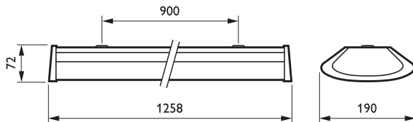
TCS022 2xTL-D36W HF P
